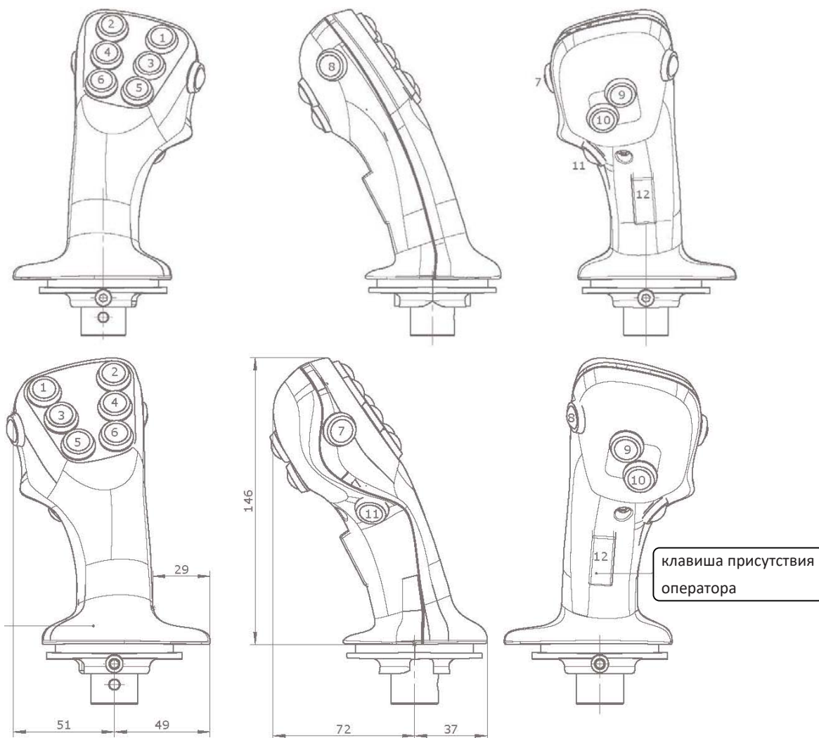
Пример исполнения конфигурации: SC-H25R-2B-2F2
